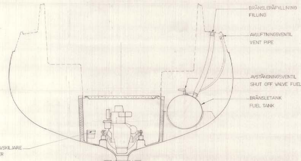
SEKTION A-A
